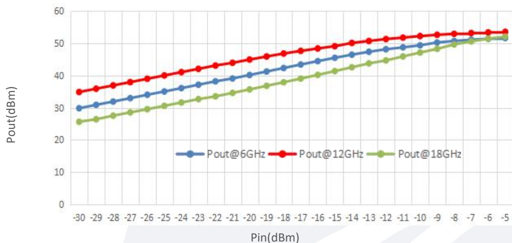
Pout@Pin
